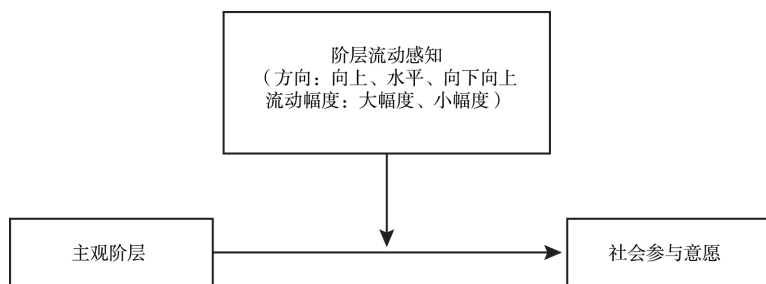
图 1 理论模型
