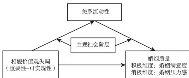
图1 变量关系
