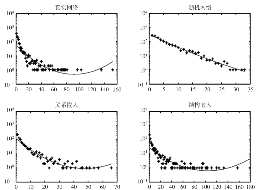
图 3 宏观层面网络指标——度分布的比较
